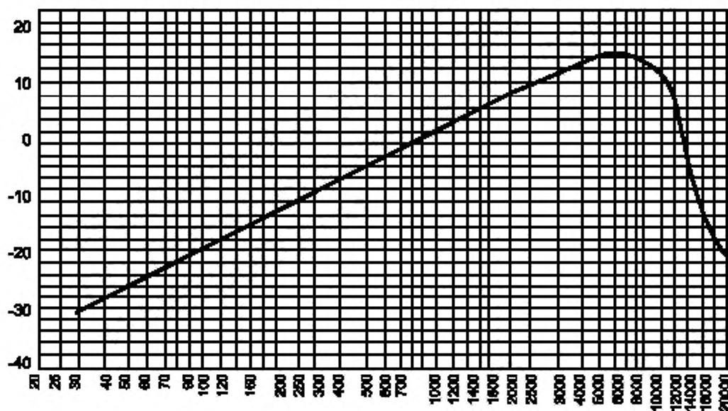
Рисунок 19 — График АЧХ псифометрического фильтра в соответствии с [1]
