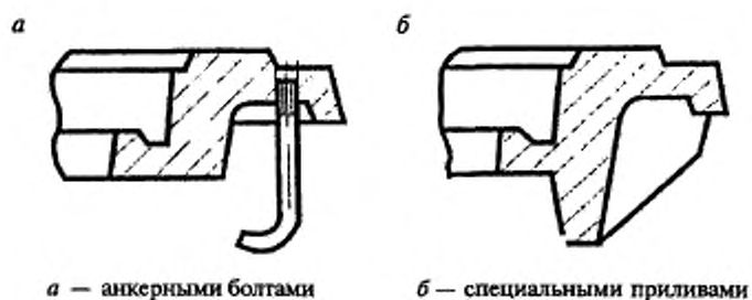
Рисунок А.4 — Усиленная заделка корпуса люка
