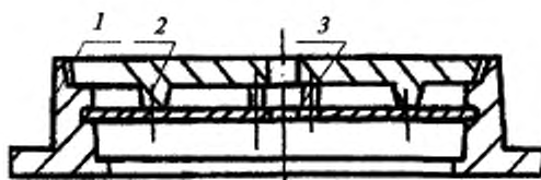
Рисунок А.2 — Люк, оснащенный запорным замковым устройством
