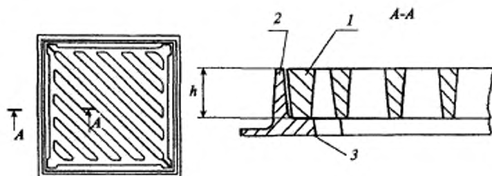
Рисунок Б.1 — Дождеприемник ливнесточного колодца
