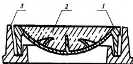
Рисунок А.2 — Люк, оснащенный запорным замковым устройством
