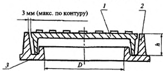
Рисунок А.1 — Люк общего назначения
