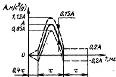
Полусинусоидальный импульс ударного воздействия
