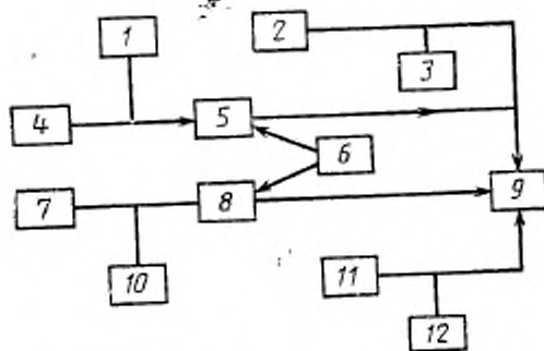
1, 3, 10, 12—вольтметры постоянного тока; 2—источник питания напряжения смещения анодов индикации; 4, 7—источники питания постоянного напряжения; 5—генератор импульсов напряжения индикации; 6—устройство управления и синхронизации; 8—генератор импульсов напряжения сканирования; 9—испытываемый индикатор; 11—источник питания напряжения анодов сканирования
