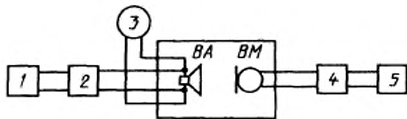
1 – генератор ГНИ; 2 – усилитель мощности У1; 3, 5 – электронный вольтметр; 4 – микрофонный усилитель УМ; BA – контролируемый громкоговоритель; BM – измерительный микрофон
