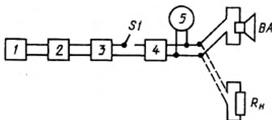
1 – генератор белого или розового шума; 2 – фильтр ФПШМ; 3 – фильтр ФЗД; 4 – усилитель мощности У2; 5 – электронный вольтметр; BA – контролируемый громкоговоритель; R_H – ре- зистор; S_1 – прерыватель
