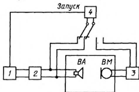
1 – генератор импульсов; 2 – усилитель мощности У1; 3 – микрофонный усилитель УМ; 4 – универсальный осциллограф; BA – контролируемый громкоговоритель; BM – измерительный микрофон
