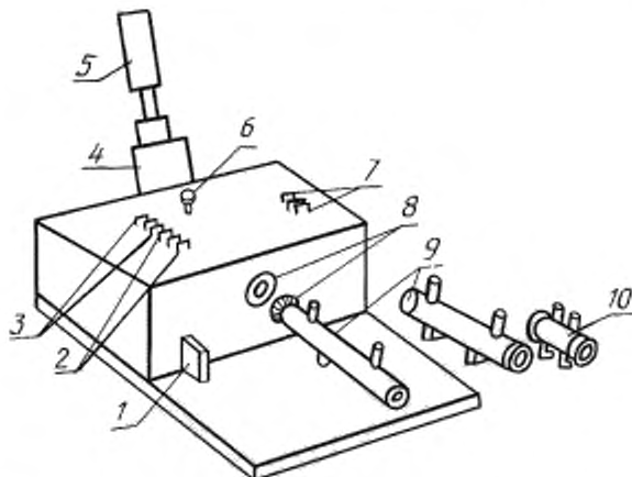
1 — кювета для масла толщиной 10 мм; 2 — набор желтых светофильтров; 3 — набор красных светофильтров; 4 — кожух с белой, рассеивающей свет, поверхностью экрана; 5 — окуляр; 6 — ручка перемещения клина; 7 — набор нейтральных светофильтров; 8 — верхнее и нижнее окна прибора; 9 — кювета для масла толщиной 130 мм; 10 — кювета для масла толщиной 50 мм
