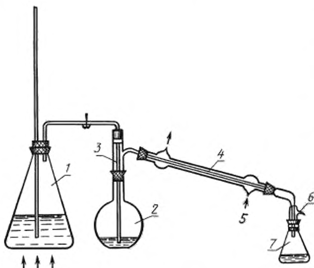
1 - паровыделитель; 2 - отгонная колба; 3 - насадка Вюрца, 4 - водяной холодильник; 5 - аплонж с отводом, 6 - регулятор давления, 7 - приемная колба
