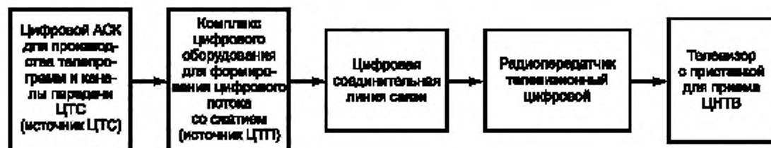
Рисунок Б.1 — Структурная схема типового тракта наземного цифрового телевидения (ЦПТВ)
