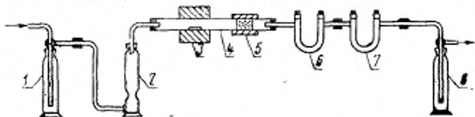
1 и 2—промывные склянки с силикагелем; 3—колонка осушения воздуха с перхлоратом магния или хлористым кальцием; 3 и 4—электрические трубчатые печи; 5—трубка сгоревшая кварцевая или фарфоровая с внутренним диаметром от 18 до 20 мм и длиной 500 мм. В зоне печи 4 трубка заполнена смесью, состоящей из окиси и двуокиси свинца и обожженной пемзы в разных массовых частях; 6 и 7—абсорбционные трубки, наполненные перхлоратом магния или хлористым кальцием.
