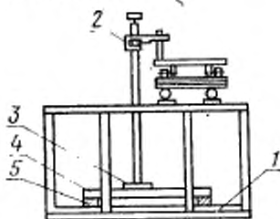
1 — плита; 2 — измеритель высоты (глубиномер); 3 — площадка для измерения высоты мягкого элемента диаметром 80 мм; 4 — испытываемый образец; 5 — брусок, применяемый при испытании образцов с гибкими, комбинированными и эластичными основаниями
