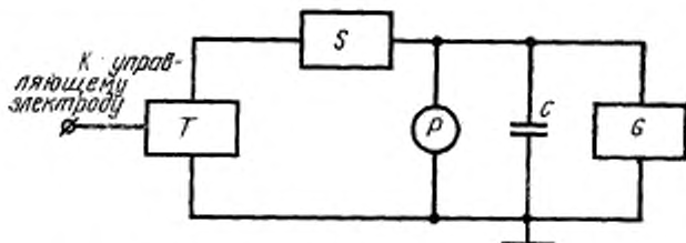
С — накопительный конденсатор; Р — измеритель напряжения; Т — импульсный трансформатор; S — коммутлирующее устройство; G — источник напряжения
