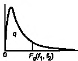
Рисунок 1 — Квантили F-распределения
