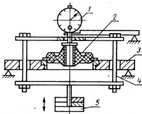
1—индикатор; 2—амортизатор; 3—опорная поверхность; 4—загрузочная рамка; 5—груз.
