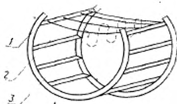
1—металлическая рама; 2—натянутые термостойкие нити; 3—испытываемая нить в свободном состоянии.
