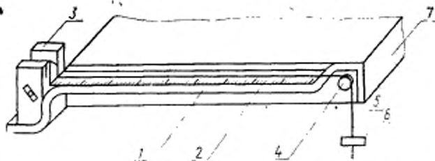
1—металлический угольник; 2—металлическая линейка; 3—зажим; 4—рама с запрессованным шарикоподшипником; 5—испытываемая нить; 6—груз предварительного натяжения; 7—рабочий стол.
