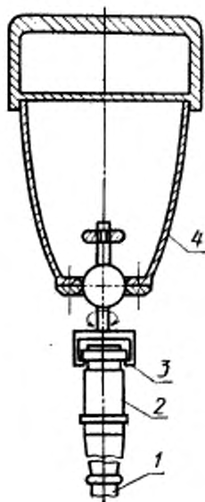
1—кабель; 2—разъем; 3—подшипники; 4—захват
