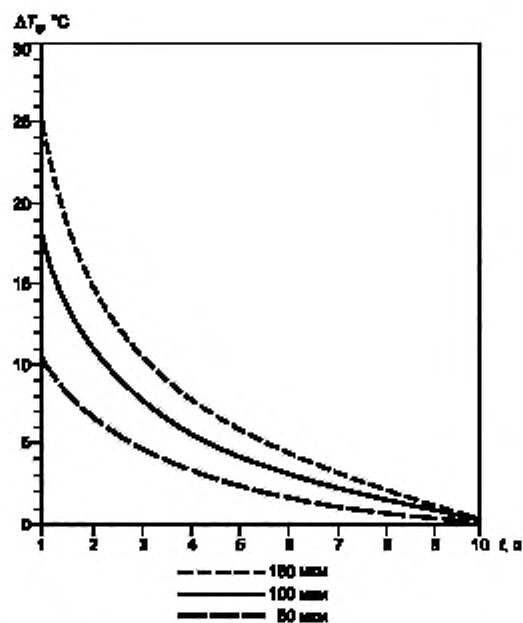
Рисунок 3а — Увеличение ожогового порога, указанного на рисунке 2, для металлической поверхности, покрытой лаком толщиной 50, 100 и 150 мкм
