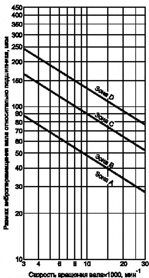
Рисунок А.1 — Рекомендуемые значения максимальных относительных перемещений вала в зависимости от максимальной рабочей скорости вращения вала агрегата
