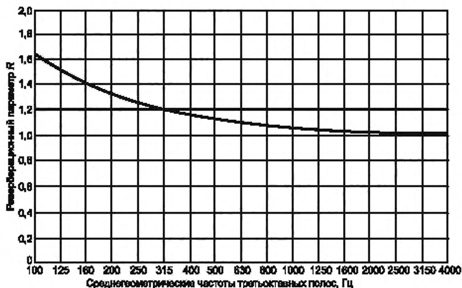
Рисунок Б.3 — Значение реверберационного параметра R для камеры объемом 70 \text{ м}^3 в функции среднегеометрической частоты третьоктавной полосы
