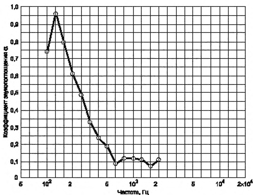
Рисунок Б.2 — Коэффициент звукопоглощения \alpha резонансного поглотителя, измеренный в реверберационной камере объемом 200 \text{ м}^3
