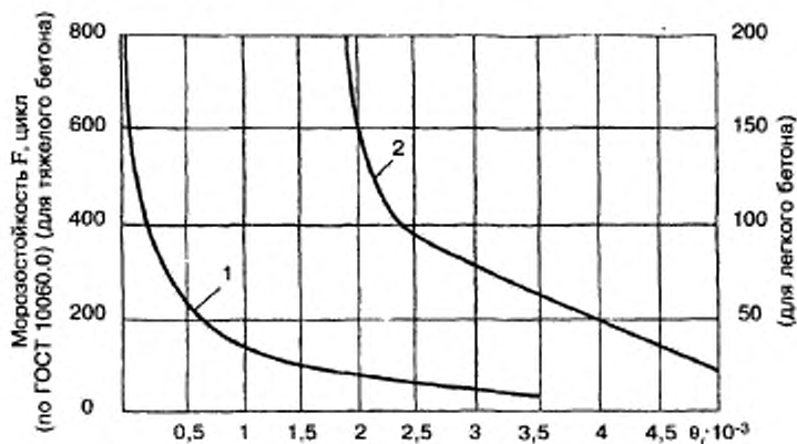
Рисунок 2 — График зависимости морозостойкости бетона от \theta , — максимального относительного увеличения разности объемных деформаций бетонного и стандартного образцов при замораживании
