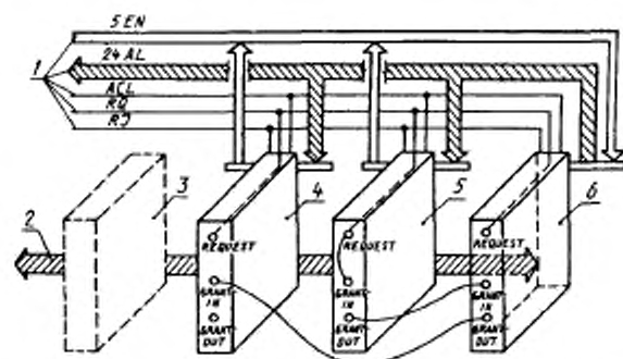
1 — линии магистрали дополнительного контроллера, 2 — магистраль крейта, 3 — модуль, 4 — дополнительный контроллер с наименьшим приоритетом, 5 — дополнительный контроллер с наибольшим приоритетом, 6 — крейт-контроллер
