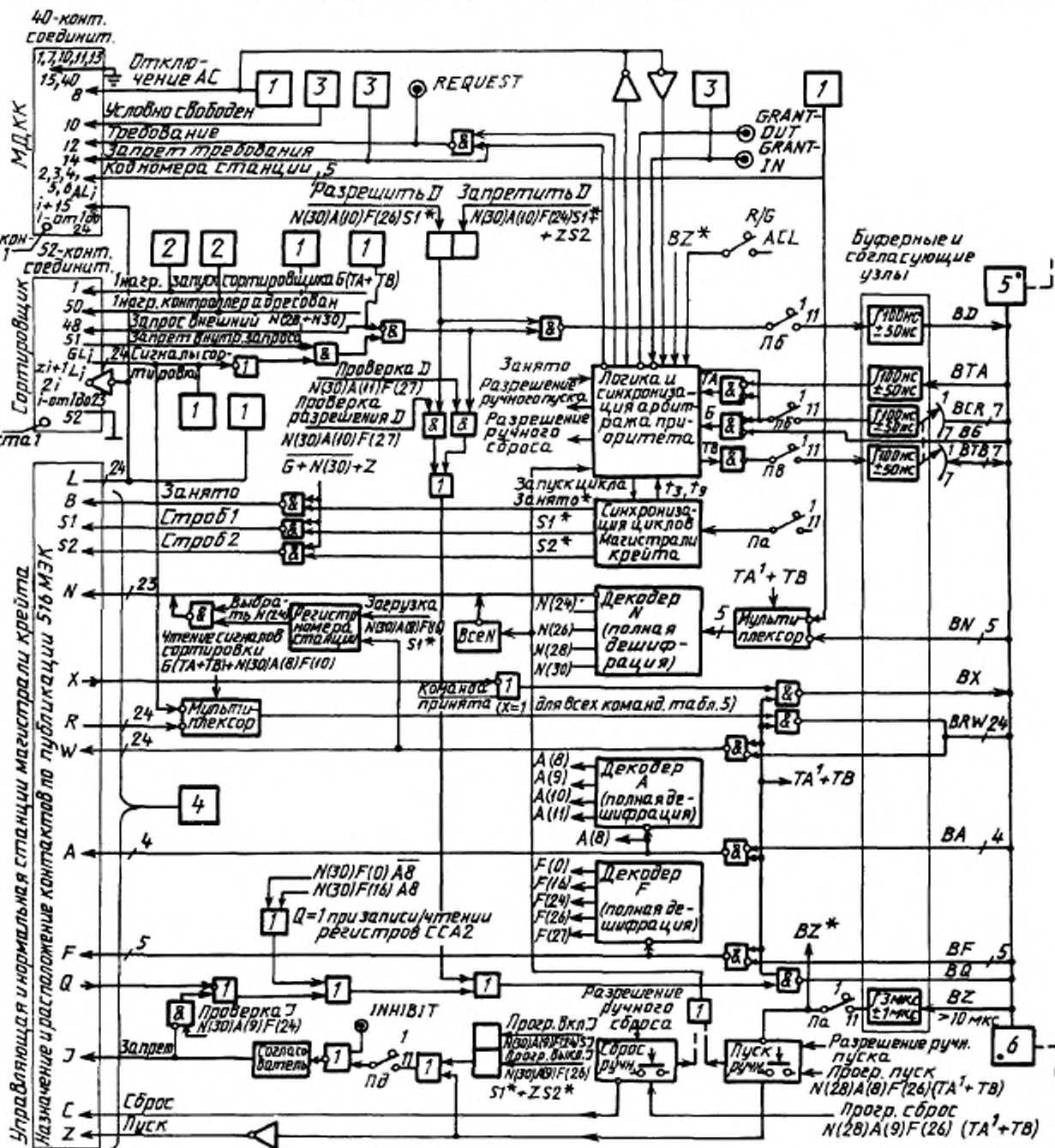
Рис. 6. К্রেйт-контроллер КАМАК типа А2 (блок двойной ширины)
