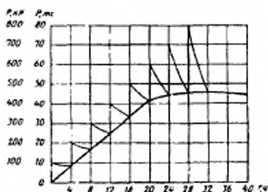
Рисунок 1 — График изменения нагрузки P во времени t
