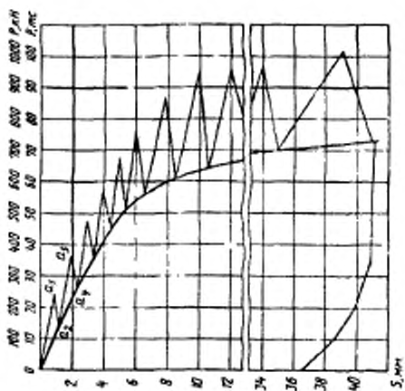
Рисунок 1 — График зависимости осадки S от нагрузки P
