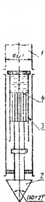
Схема конструкции сваи-зонда
