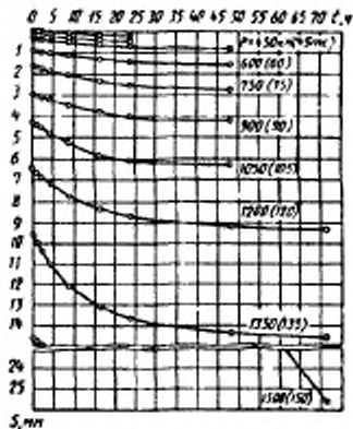
График изменения осадки сваи S во времени t (по ступеням нагрузки)
