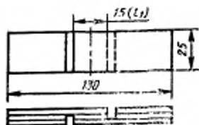
Черт. 4, лист 1
