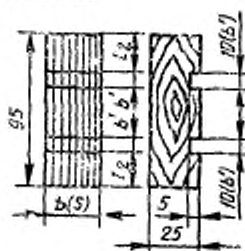
Черт. 7
