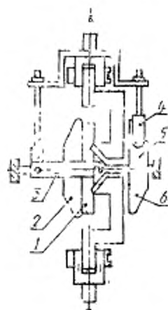
1 — образец, 2 — упорная планка, 3 — планка; 4 — захват, 5 — упор, 6 — траверса
