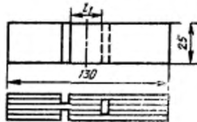
Черт. 4, лист 2
