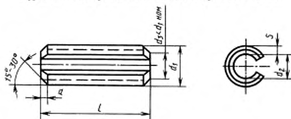
Пружинный штифт номинальным диаметром d_1 > 12 мм
