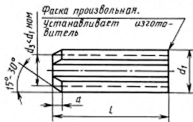
Пружинный штифт номинальным диаметром d_1 > 12 мм
