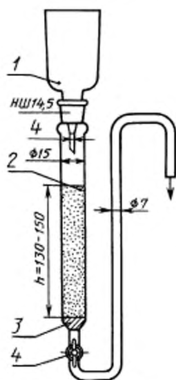
1 — резервуар вместимостью 50 см 3 ; 2 — колонка с кадмием; 3 — стеклянная вата; 4 — кран
