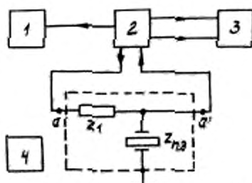
1 — частотомер; 2 — измеритель АЧХ; 3 — графопостроитель; Z_{н.э} — проверяемый ПЭП; Z_1 — электрическая нагрузка; 4 — акустическая нагрузка
