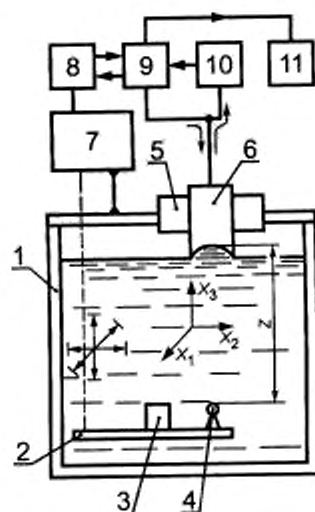
1 — иммерсионная ванна; 2 — узел фиксации отражателя; 3 — плоский отражатель; 4 — сферический отражатель; 5 — узел фиксации ПЭП; 6 — проверяемый ПЭП; 7 — механизм перемещения по координатам X_1 , X_2 , X_3 ; 8 — графопостроитель; 9 — приемник; 10 — генератор радиомпульсов; 11 — осциллограф
