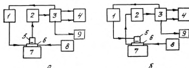
1 — усилитель мощности; 2 — усилитель напряжения (черт. 40а), усилитель тока (черт. 40б); 3 — измеритель АЧХ; 4 — графопостроитель; 5 — проверяемый ПЭП; 6 — диэлектрический преобразователь; 7 — акустическая нагрузка; 8 — источник напряжения; 9 — частотомер
