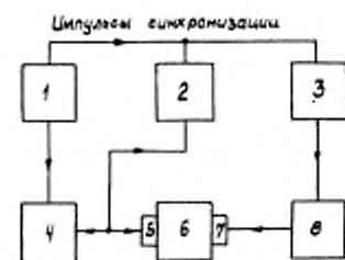
1, 3 — генераторы импульсов; 2 — осциллограф; 4, 8 — электронные блоки УПНК; 5 — проверяемый ПЭП; 6 — стандартный образец; 7 — вспомогательный ПЭП
