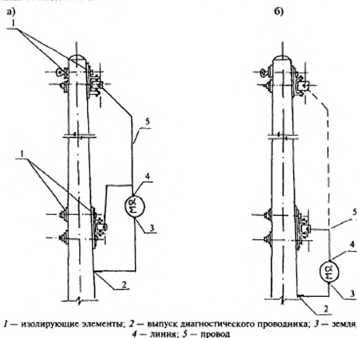
Рисунок 3 — Схема измерения электрического сопротивления между деталями для крепления консолей и кронштейнов и арматурой а — полного сопротивления; б — сопротивления одной детали
