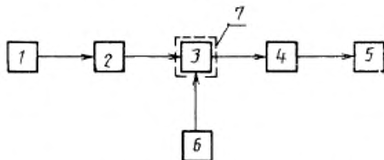
1—источник излучения; 2—модулятор; 3—испытуемый ФЭПП (ФПУ); 4—усилительное устройство; 5—регистрирующий прибор, 6—источник питания; 7—камера тепла и холода
