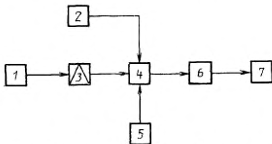
1 — источник излучения; 2 — источник фонового излучения; 3 — модулятор; 4 — испытуемый ФЭПП (ФПУ); 5 — источник питания ФЭПП (ФПУ); 6 — усилительное устройство; 7 — регистрирующий прибор
