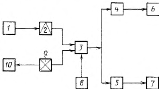
1—источник излучения; 2—модулятор; 3—непылеемый ФЭПП (ФПУ); 4—усилительное устройство измерения напряжения (тока) шума; 5—усилительное устройство измерения напряжения (тока) фотосигнала; 6—регистрирующий прибор для измерения напряжения (тока) шума; 7—регистрирующий прибор для измерения напряжения (тока) фотосигнала; 8—источник питания ФЭПП (ФПУ); 9—система охлаждения; 10—датчик моментов включения и выключения системы охлаждения.
