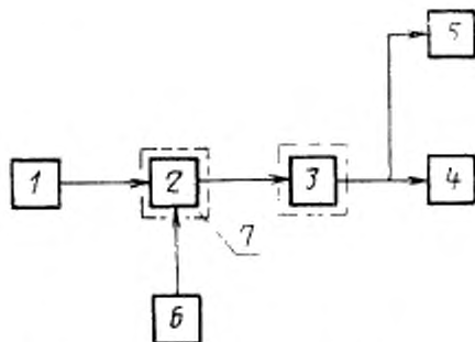
1—источник визуального излучения, 2—испытываемый ФЭПП (ФПУ); 3—усиливающее устройство; 4—регистрирующий прибор для измерения напряжения (тока) фотосигнала; 5—регистрирующий прибор для измерения напряжения (тока) шума, 6—источник питания; 7—камера тепла и холода
