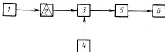
1 — источник излучения; 2 — модулятор; 3 — испытываемый ФЭПП (ФПУ); 4 — источник питания ФЭПП (ФПУ); 5 — усилительное устройство; 6 — регистрирующий прибор
