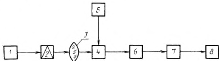
1—источник излучения; 2—модулятор; 3—оптическая система; 4—испытуемый ФЭПП (ФПУ); 5—координатный столик; 6—коммутатор; 7—усилительное устройство; 8—регистрирующий прибор
