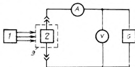
1 — источник излучения; 2 — испытуемый ФЭПП; А — измеритель тока; В — измеритель напряжения; G — источник питания, Э — светозащитный экран
