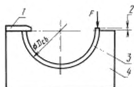
Контрольный блок
