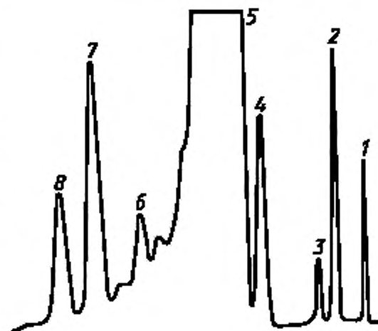
Типовая хроматограмма
