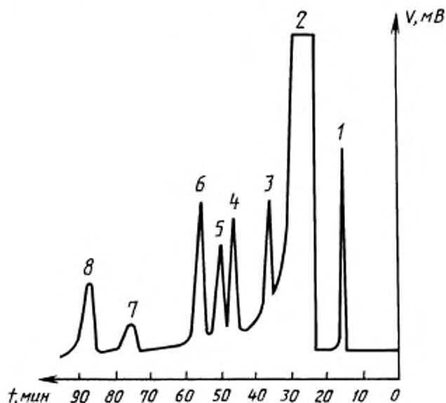
Типовая хроматограмма искусственной смеси четыреххлористого углерода и хлорорганических примесей на колонке с насадкой 1
