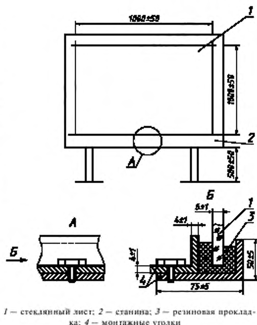
Рисунок 2 — Схема закрепления стеклянного листа
