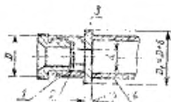
1 — гнездо; 2 — шайба; 3 — кольцо, 4 — труба
