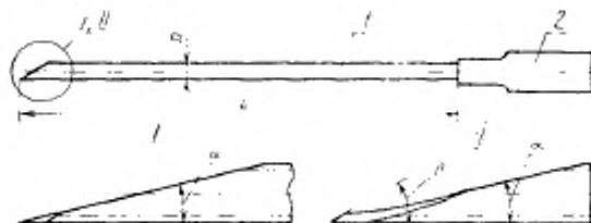
1—головка; 2—труба Черт. 1
