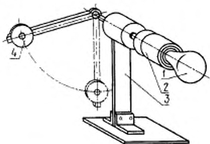
1—лампа; 2—патрон; 3—стойка; 4—противовес
