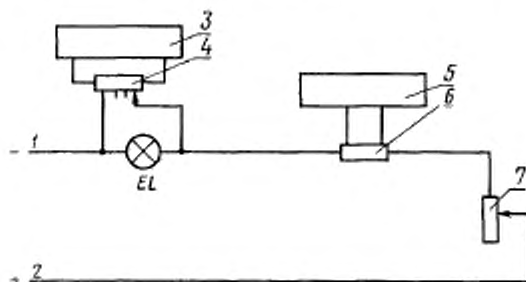
1, 2—выводы для подключения к источнику питания; 3, 5—потенциометры для измерения напряжения и силы тока в лампе; 4—делитель напряжения; 6—образцовая катушка сопротивлений; 7—регулируемый реостат; EL—измеряемая или образцовая светоизмерительная лампа
