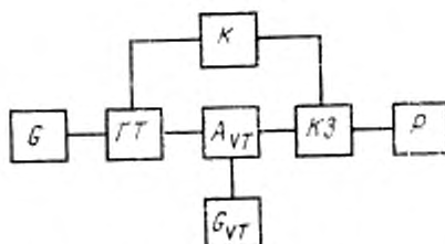
Схема измерения |h'_{21б}| , |h'_{21э}| или \arg(h'_{21б})
