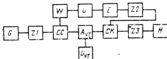
Схема измерения |h_{212}| или \arg(h_{216}) при отсутствии генератора тока во входной цепи проверяемого транзистора и компенсации сигнала в выходной цепи
