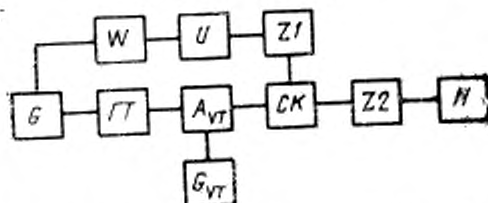
Схема измерения |h_{212}| или \arg(h_{216}) компенсационным способом
