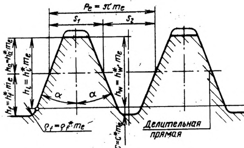
Пара исходных контуров
