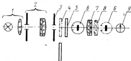
1 — осветитель; 2 — коллиматор; 3 — ирисовая диафрагма; 4 — прозрачный экран; 5 — светофильтр; 6 — фотоприемник; 7 — испытуемый объектив; 8 — вспомогательная оптическая система; 9 — измерительный прибор
