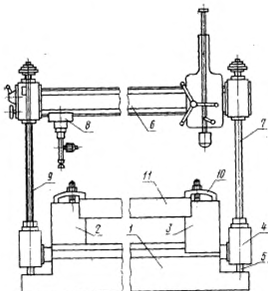
1—основание машины; 2—неподвижная опора; 3—подвижная опора; 4—каретка; 5—направляющая каретки; 6—траверса; 7—ходовка для перемещения траверсы; 8—датчик сил; 9—измеритель перемещений; 10—прижимы; 11—испытуемое изделие.
