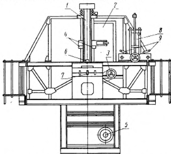
1—стойка; 2—испытуемое изделие; 3—привод; 4—рычаги-толкатели; 5—гидробак; 6—счетчик оборотов; 7—пульт управления; 8—нагружающее устройство; 9—сигнальное устройство.
