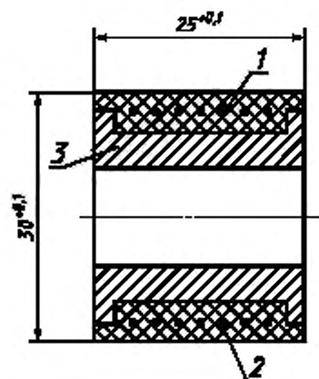
1 — покрытие из токопроводящей резины; 2 — проводочный бандаж; 3 — латунная втулка
