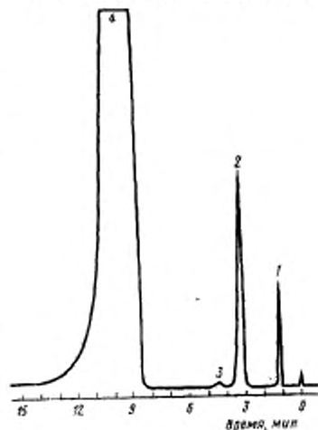
1 — гексан „внутренний эталон“; 2 — бензол; 3 — изопропиловый спирт; 4 — 1,4-диоксан
