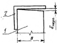
1—панель; 2—поверочный угольник 90^\circ ; В—ширина панели
