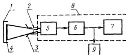
1—световой шкаф; 2—светофильтры; 3—тубус; 4—испытательная таблица; 5—телевизионная камера; 6—приборы в составе ПТУ; 7—видеоконтрольное устройство; 8—ПТУ; 9—осциллограф
