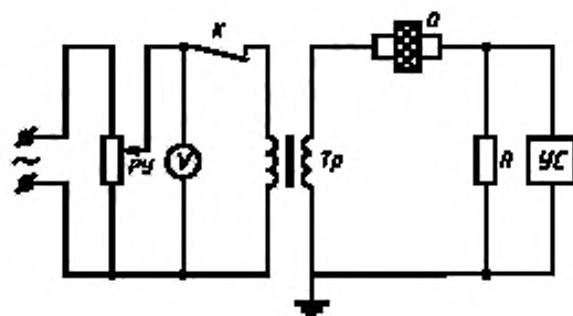
Tr — высоковольтный испытательный трансформатор; R — резистор; PУ — регулятор напряжения; O — образец с электродами; V — вольтметр для измерения напряжения пробоя; ВУ — выпрямительное устройство; C — конденсатор; УС — устройство сигнализации о наступлении пробоя; K — контакт устройства сигнализации, отключающий первичную цепь трансформатора в момент пробоя образца
