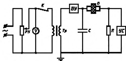
Tr — высоковольтный испытательный трансформатор; R — резистор; PУ — регулятор напряжения; O — образец с электродами; V — вольтметр для измерения напряжения пробоя; УС — устройство сигнализации о наступлении пробоя; K — контакт устройства сигнализации, отключающий первичную цепь трансформатора в момент пробоя образца
