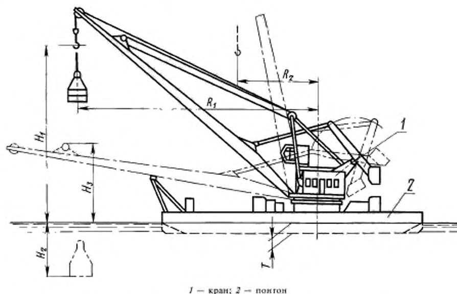
1 — кран; 2 — понтон
