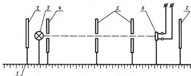
1 — скамья; 2 — концевые экраны; 3 — источник излучения; 4 — диафрагма; 5 — промежуточные диафрагмы; 6 — приемник излучения
