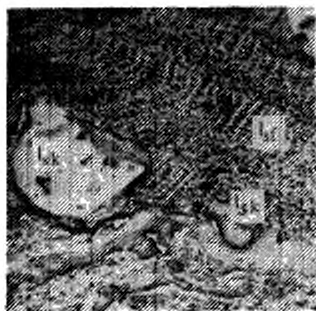
Отраженный свет 100 \times I 2f — семифоизинит I 2sk — склеротинит Черт. 7
