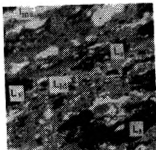
Отраженный свет Масляная иммерсия 400 \times L s - споринит L ma - макринит L sd - диктодеринит Черт. 9
