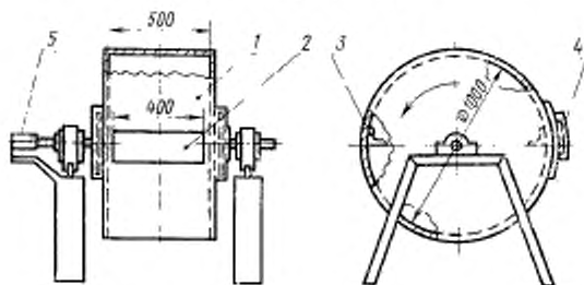
1—барaban; 2—загрузочный люк; 3—уголки; 4—крышка люка; 5—счетчик оборотов
