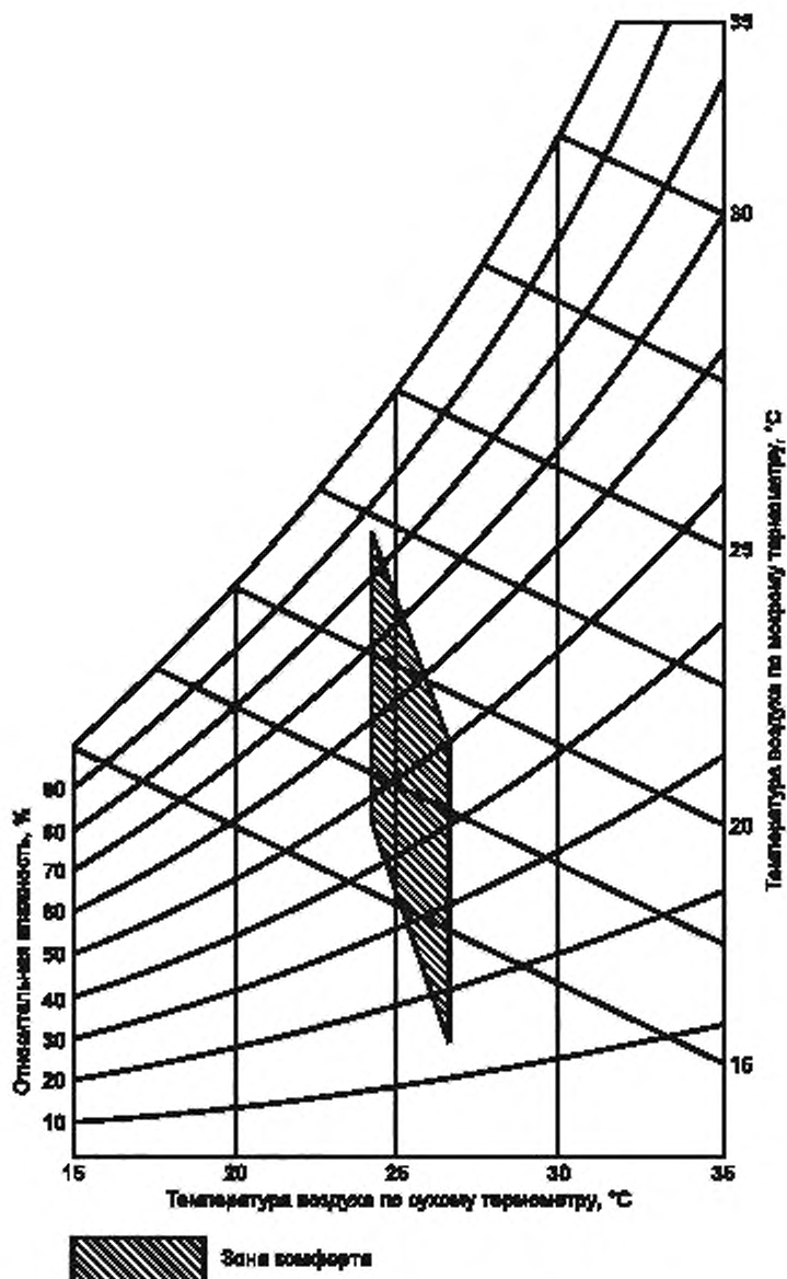
Рисунок 1 — Диаграмма эффективных температур
