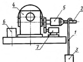
1 — образец провода; 2 — стержень; 3 — нагрузка; 4 — электродвигатель; 5 — вращающийся зажим; 6 — пусковое устройство; 7 — счетчик числа витков
