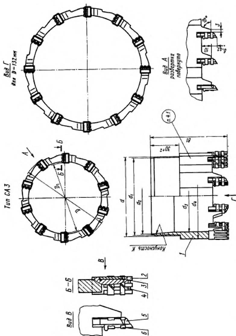
1—корпус коронки; 2—пластинка твердосплавная по документации, установленной в установленном порядке; 3—пластинка твердосплавная по ГОСТ 880—67; 4—пластина установочная; 5—пластина обортная; 6—пластина обортная.
