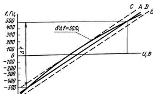
Модуляционная характеристика управляемого напряжением кварцевого генератора
