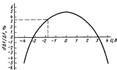
График нелинейности модуляционной характеристики управляемого напряжением кварцевого генератора
